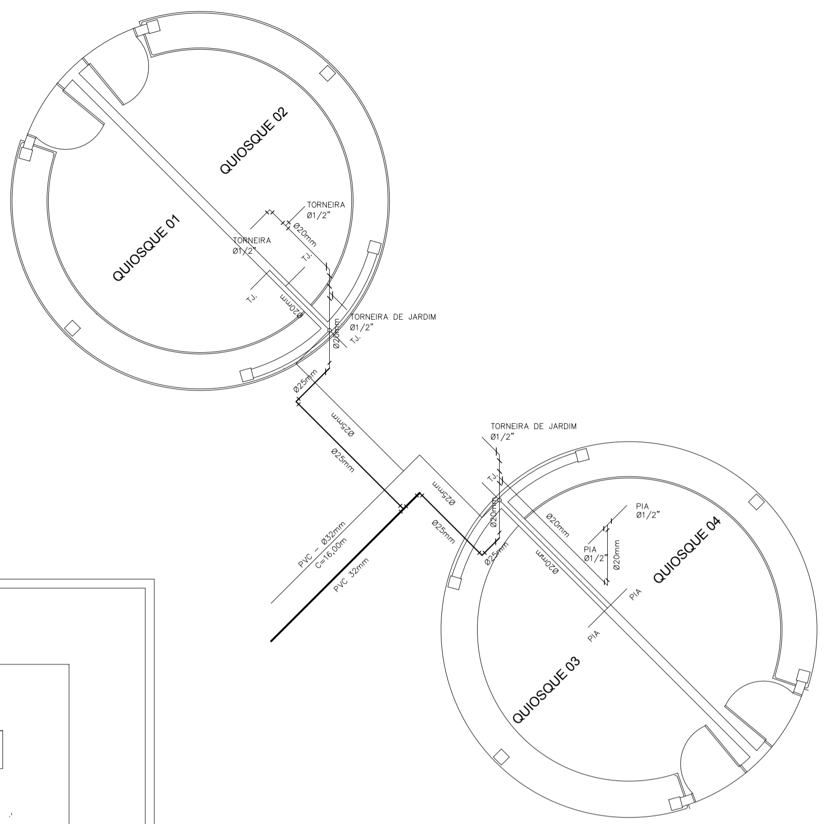
ISOMETRICO - QUIOSQUES ESC.: 1/50.
