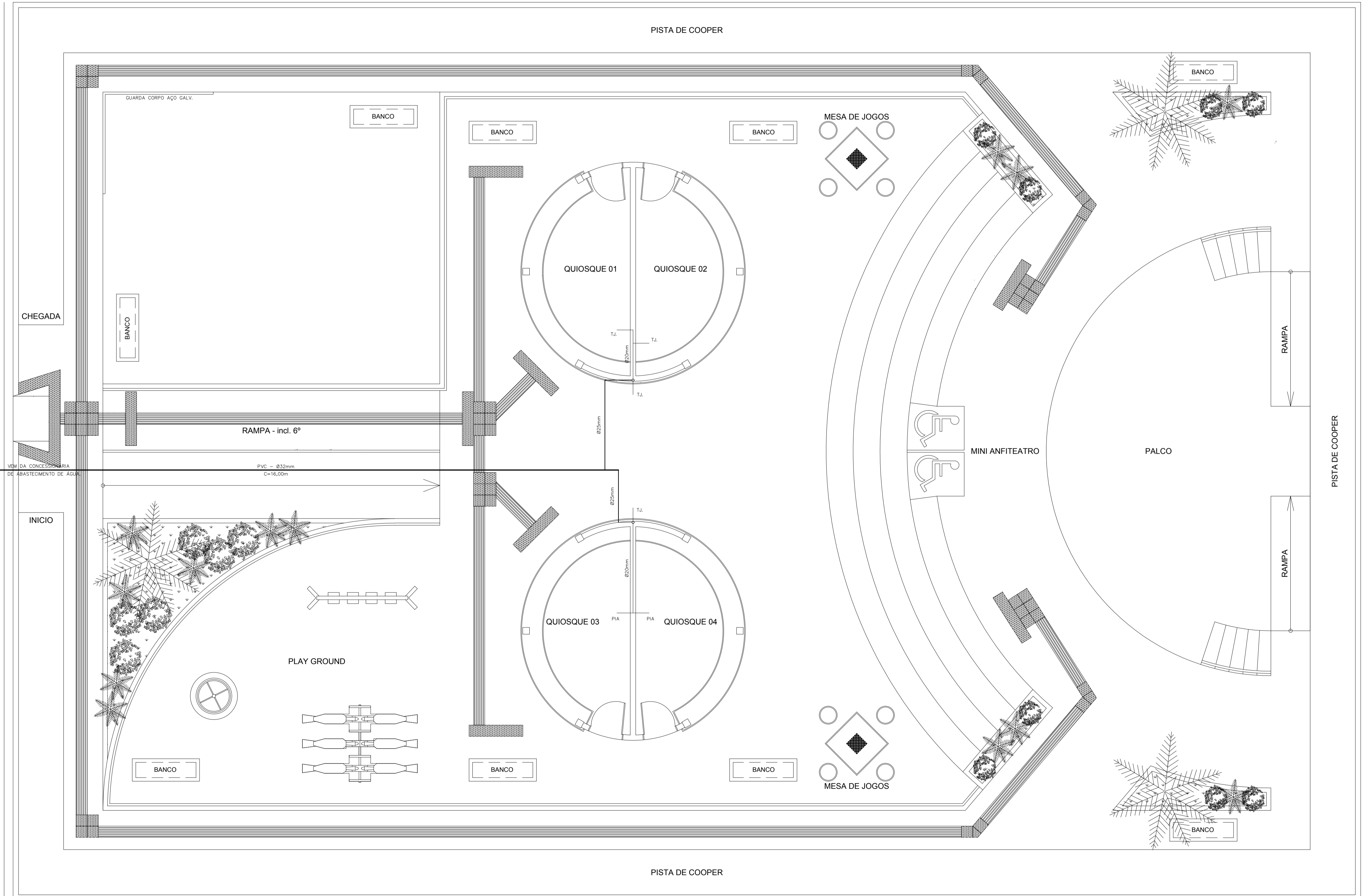
PLANTA BAIXA - IMPLANTAÇÃO ESC.: 1/50
